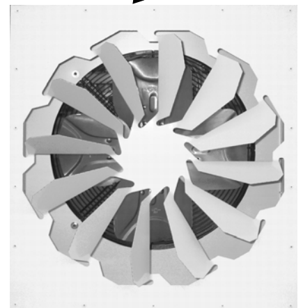
3 - Ventilátor lapátok nyitott állásban
