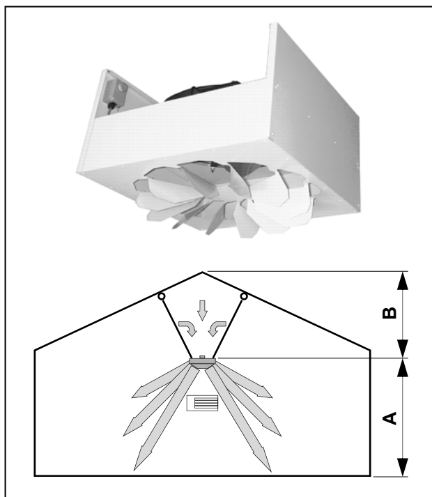
A berendezéseket a magasság 2/3 nál kell függeszteni.
